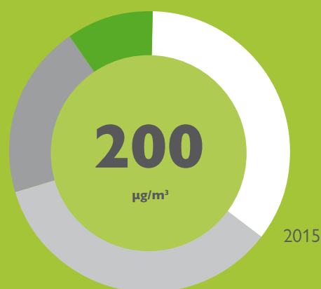
Figura 9 – Composizione di un carico estivo di ozono di 200 \mu g/m^3
