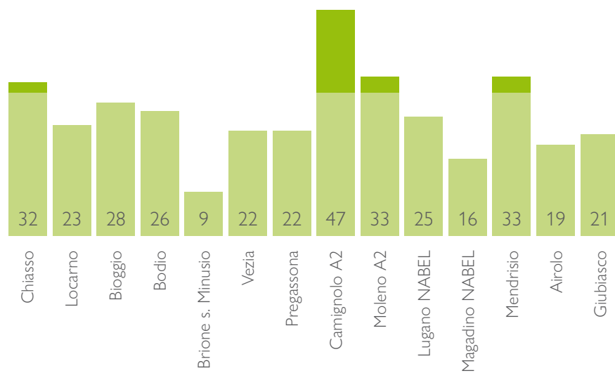
Figura 4 – Medie annue di diossido di azoto nel 2018, in \mu\text{g}/\text{m}^3
