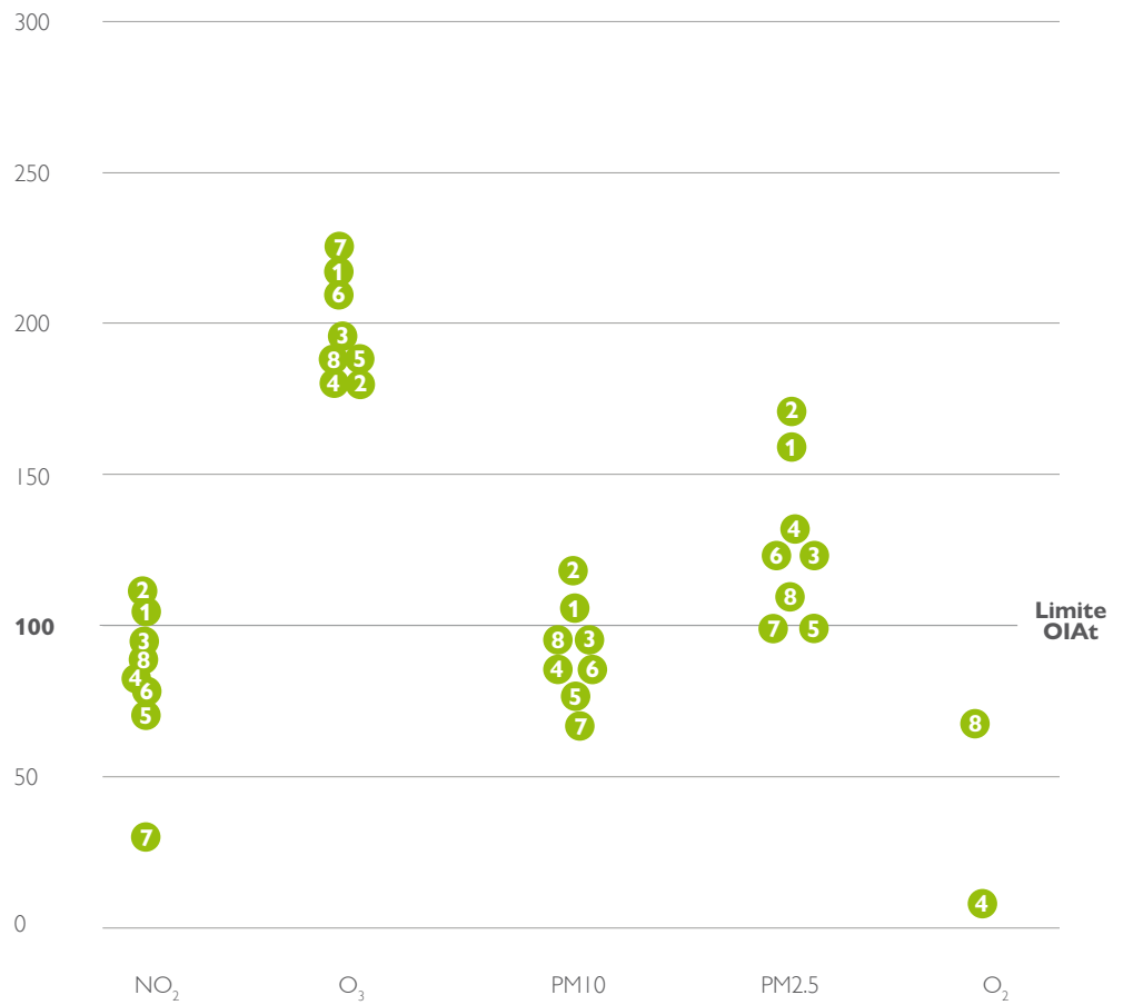
Figura 3 – Percentuale di conformità all'OIAt
