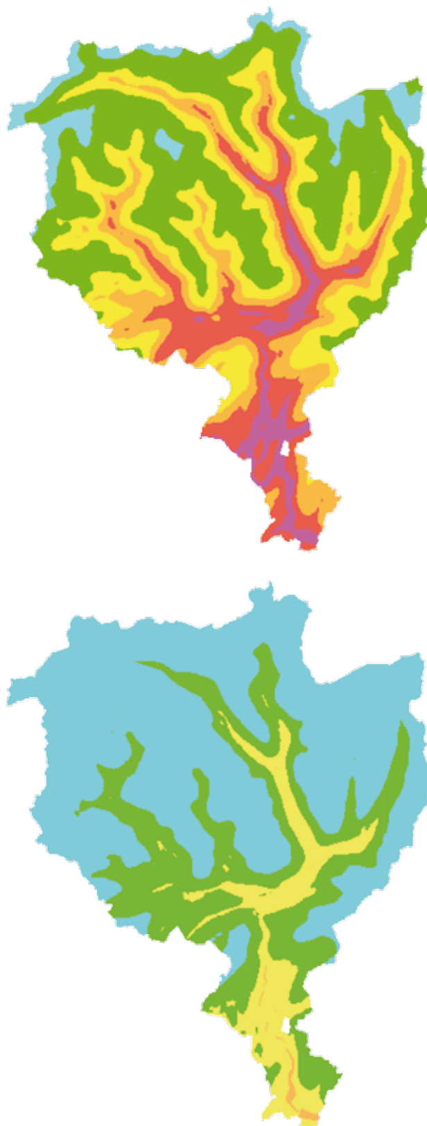
Figura 14 – Immissioni di PM10 in Ticino nel 1998 (sopra) e 2018 (sotto)
