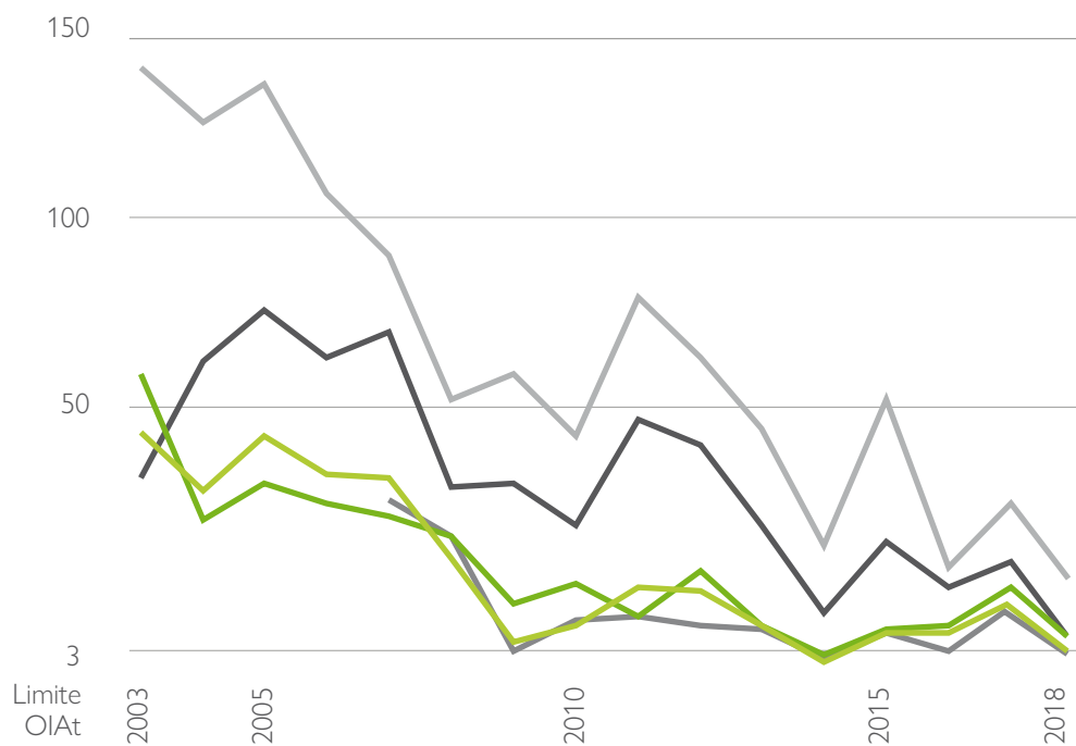
Figura 13 – Evoluzione del numero di superamenti del limite giornaliero
