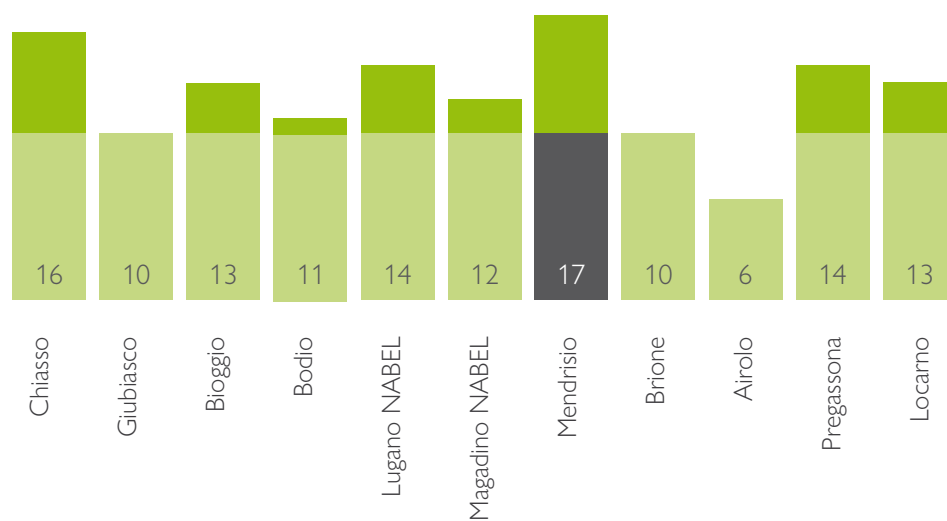
Figura 11 – Medie annue delle PM2.5 nel 2018, in \mu\text{g}/\text{m}^3
