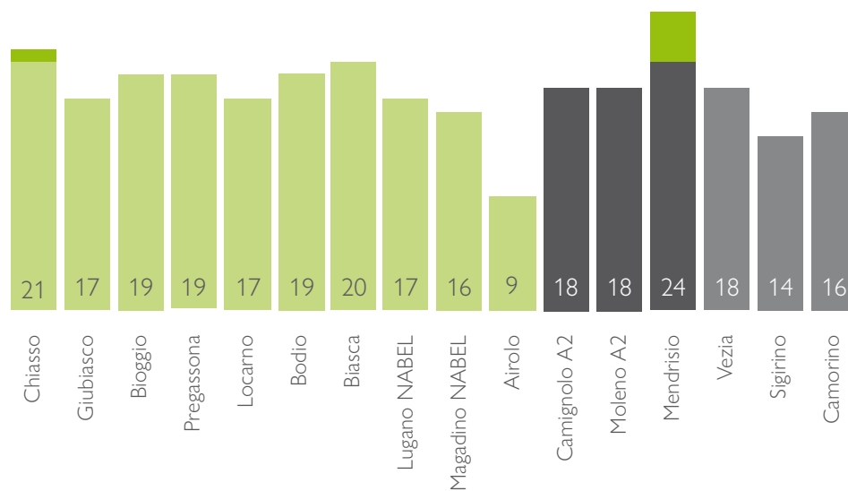
Figura 10 – Medie annue delle PM10 nel 2018, in \mu\text{g}/\text{m}^3
