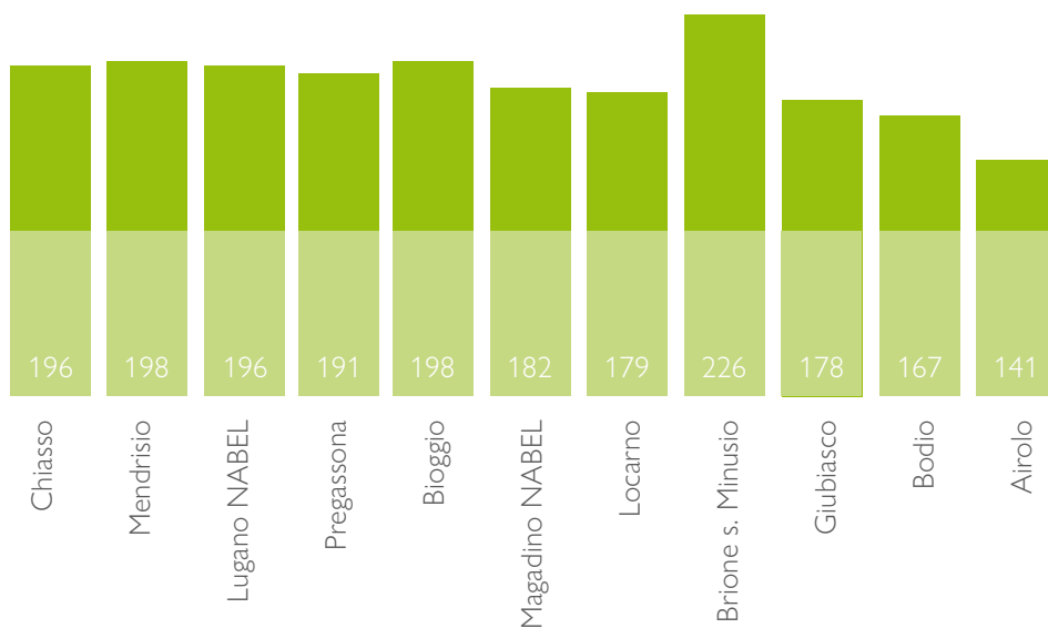
Figura 7 – 98° percentile mensile massimo di ozono nel 2018
