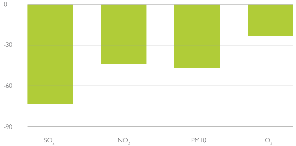
Figura 2 – Variazione percentuale delle immissioni (1990–2018)
